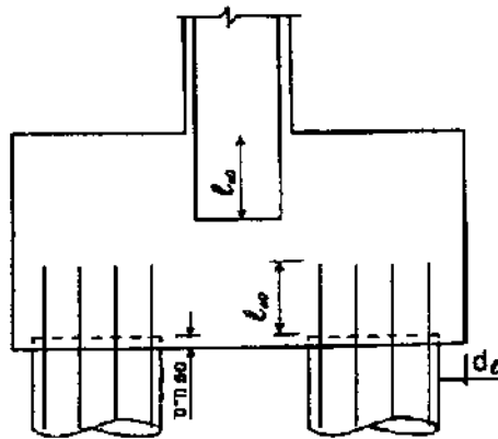
ציור 31.9 – ראש קבוצת כלונסאות - חסמחת אורכי עיגון (חמידה במילימטרים)
